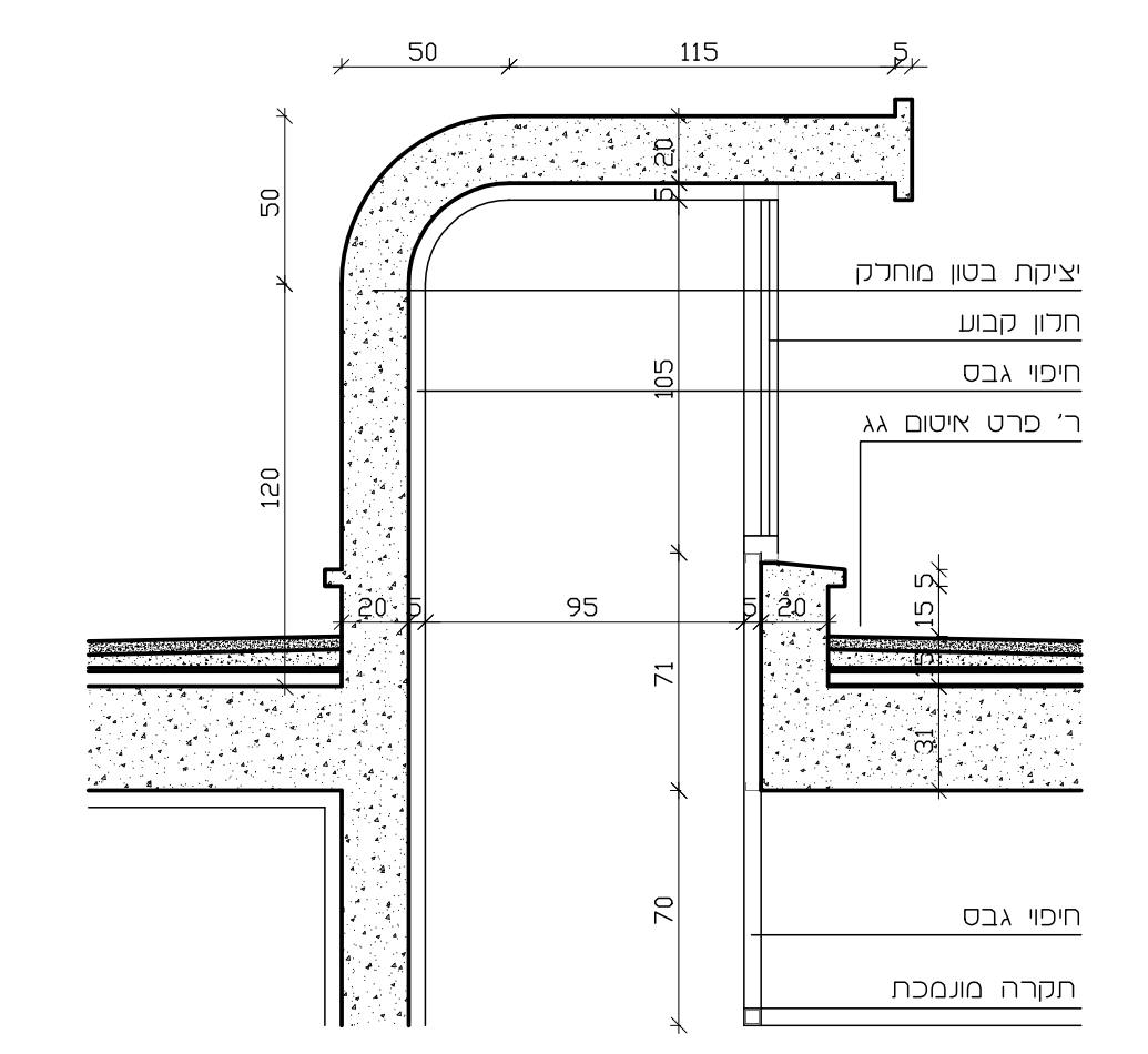
פרט SKYLIGHT עליון P07
