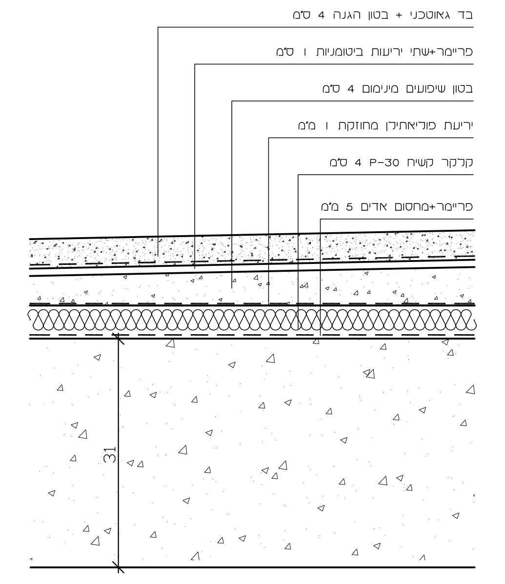
פרט איטום גג עליון P06
