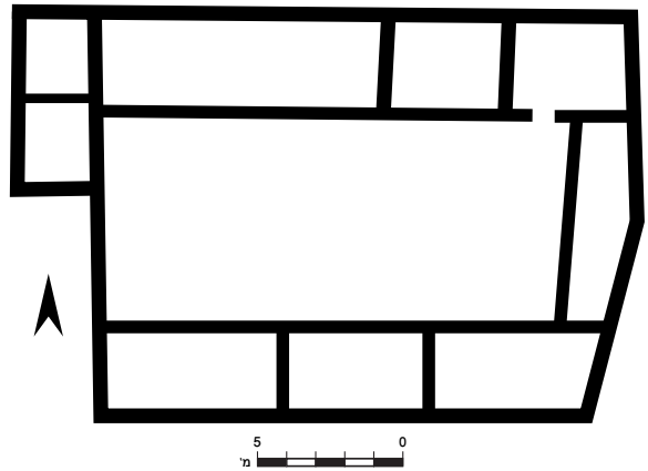
איור 5. תכנית המצודה בהר עצמון.
